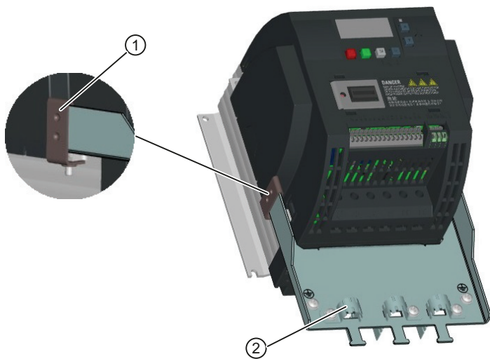
对于穿墙式安装的变频器：
