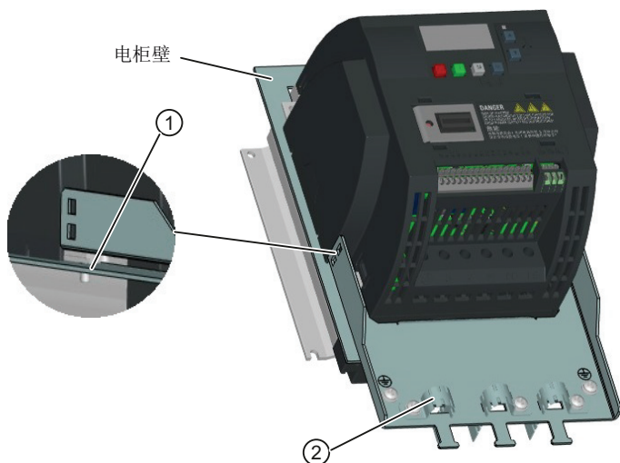
变频器外形尺寸 B / C / D
