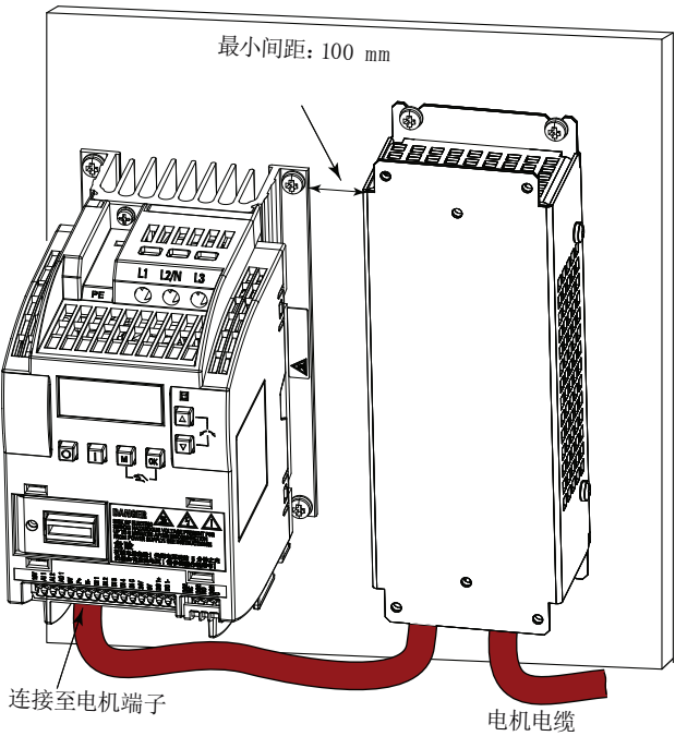
连接输出电抗器到变频器
